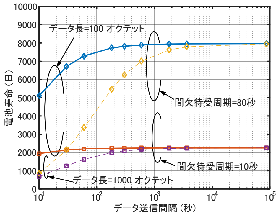
電池寿命の試算
